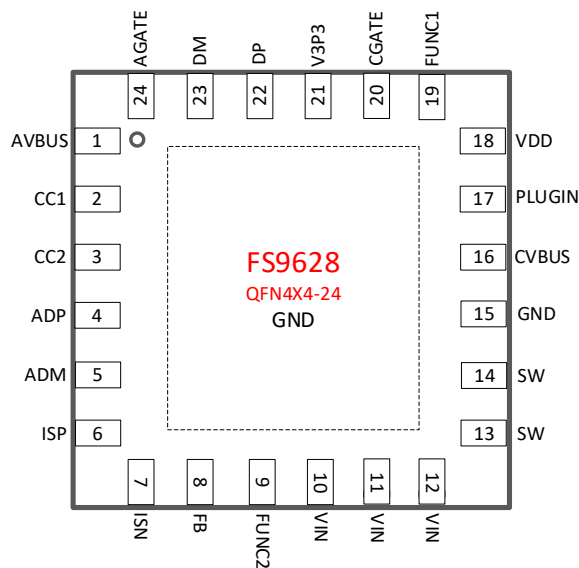
图 1. 引脚定义
