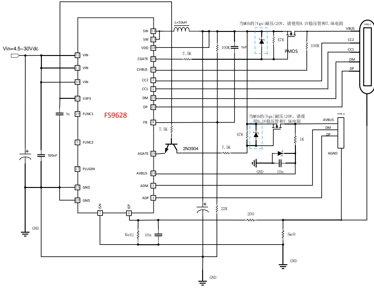
FS9628H应用图
