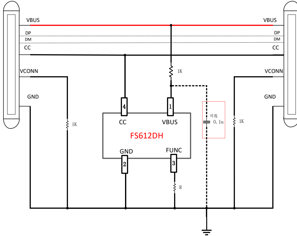
FS612DH应用图
