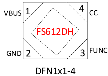
图 1.引脚定义
