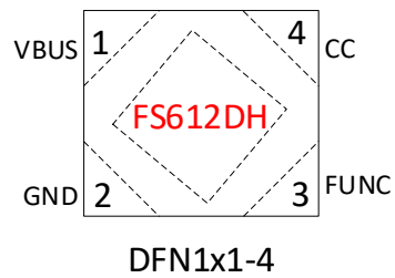
图 1.引脚定义
