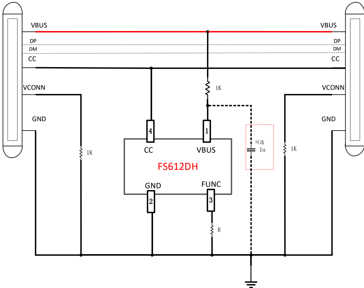
FS612DH应用图
