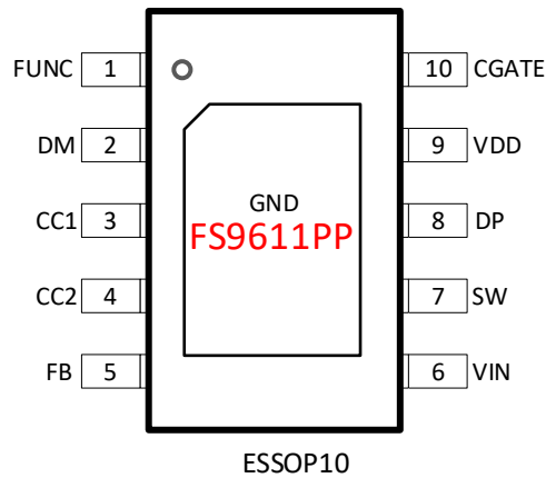
图 1. 引脚定义
